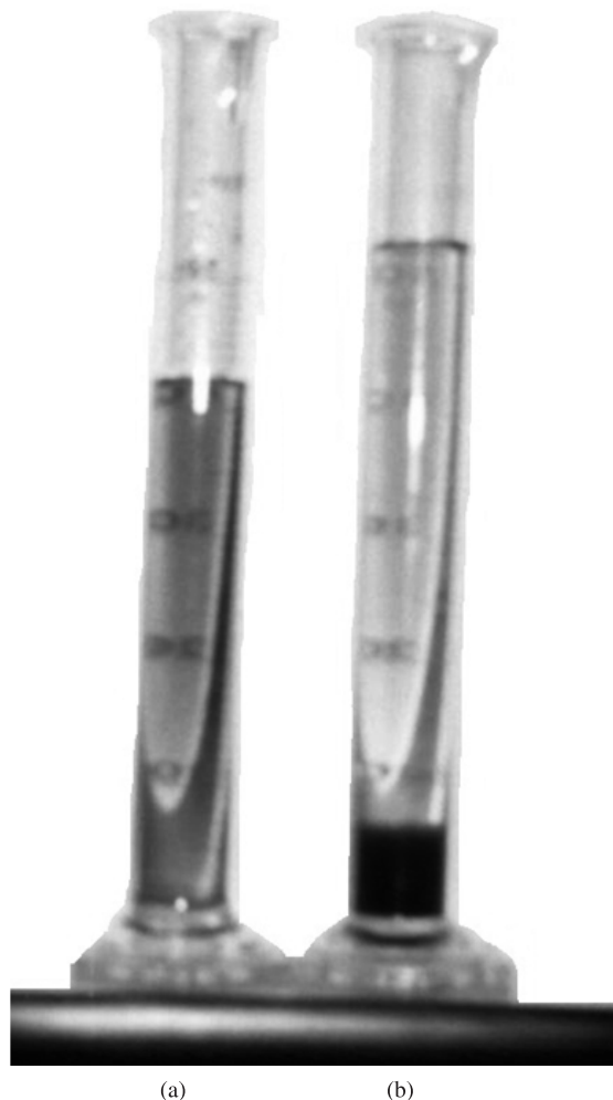
Figura 7. Teste de sedimentação a) antes, e b) após a adição do sulfato de alumínio.
