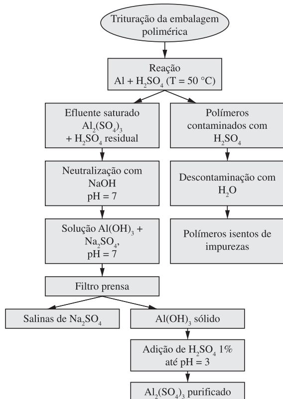
Figura 1. Fluxograma ilustrativo do processo de reciclagem.
