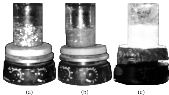
Figura 3. Desenvolvimento da reação 1, entre o ácido sulfúrico e o alumínio, a) início entre 0 a 5 minutos, b) extração entre 5 a 12 minutos, e c) final com todo alumínio dissolvido.
