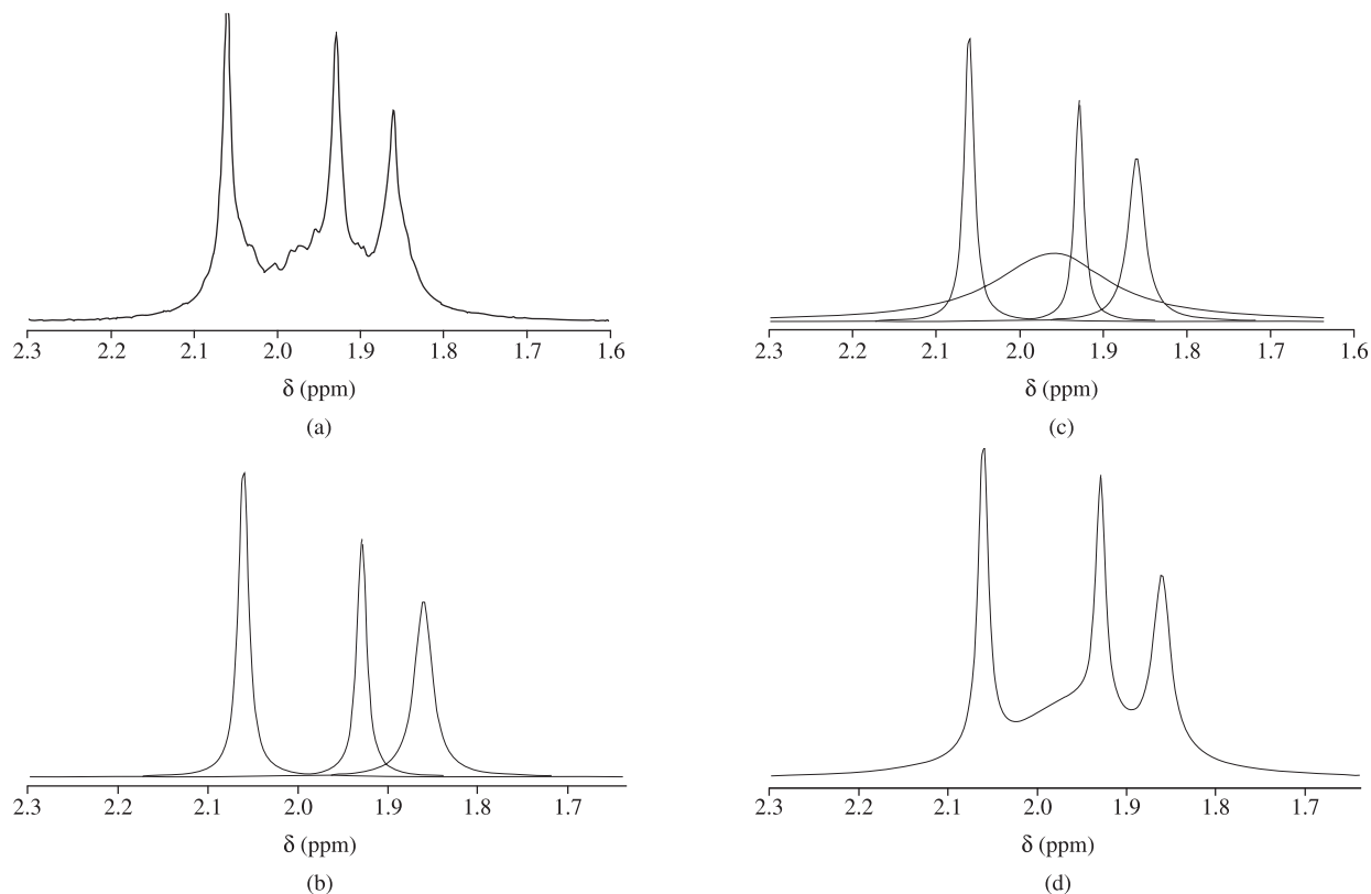
Figura 3. Sequência de deconvolução para a região correspondente aos sinais do grupo metila no espectro de 1 H-RMN do diacetato de celulose. a) espectro original; b) adição dos sinais principais; c) adição do sinal secundário; d) somatório das curvas de deconvolução.
