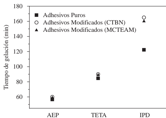
Figura 3. Tiempo de gelación determinado a 40 °C a partir de los análisis reológicos para los adhesivos puros (■) y para los adhesivos con 10 phr de cada modificador. CTBN: copolímero derivado del butadieno (○); y MCTEAM: copolímero acrílico (▲).
