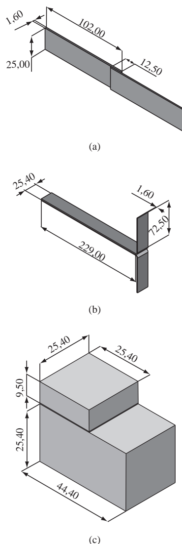
Figura 1. Geometría y dimensiones de las uniones adhesivas de acero-acero (medidas en mm). a) unión de simple sobreposición; b) unión de pelado en T; y c) unión de impacto.
