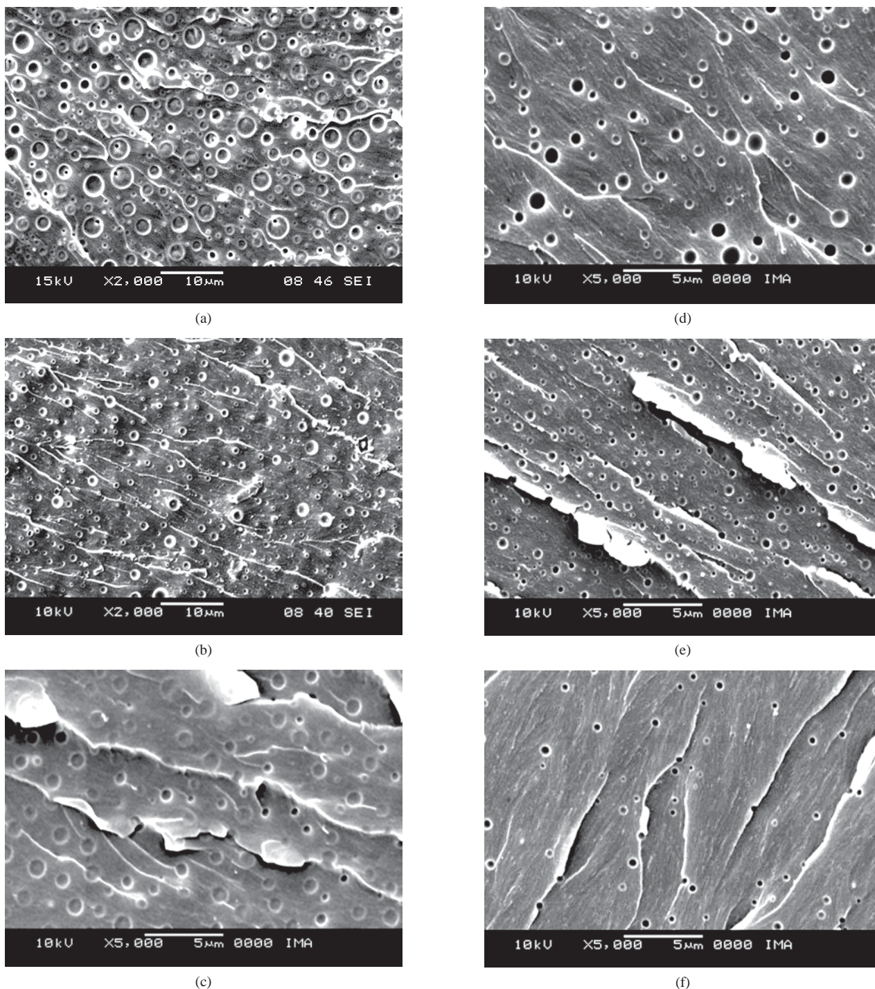
Figura 5. Micrografías electrónicas (SEM) de la superficie de fractura de los adhesivos modificados después del programa de curado. a) DGEBA/CTBN/TETA; b) DGEBA/MCTEAM/TETA; c) DGEBA/CTBN/AEP; d) DGEBA/MCTEAM/AEP; e) DGEBA/CTBN/IPD; e f) DGEBA/MCTEAM/IPD.
