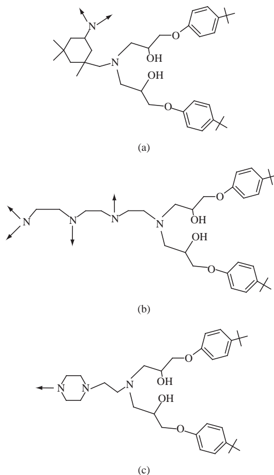
Figura 6. a) estructuras químicas de las redes epoxídicas generadas por el curado de la resina del tipo a) DGEBA con isofofondiamina (IPD); b) con trietilentetramina (TETA); y c) con N-(2-aminoetil)piperazina (AEP).
