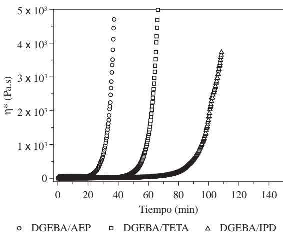
Figura 2. Evolución de la viscosidad compleja ( \eta^* ) de los adhesivos puros analizados como una función del tiempo en condiciones isotérmicas a 40 °C.
