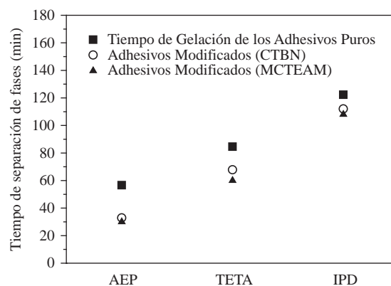
Figura 4. Tiempo de gelación para los adhesivos puros (■) y tiempo de separación de fases para los adhesivos con 10 phr de cada modificador. CTBN: copolímero derivado del butadieno (○); y MCTEAM: copolímero acrílico (▲). Determinados a partir de los análisis reológicos a 40 °C.
