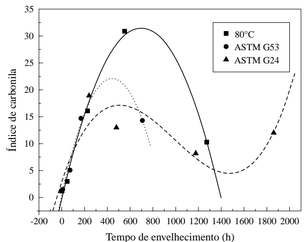
Figura 8. Tendência de variação do índice de carbonila para as três técnicas utilizadas.
